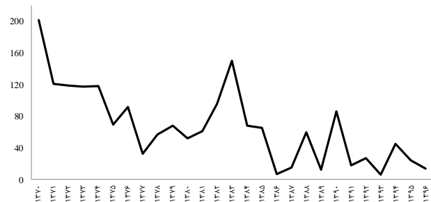
شکل ۴- دبی رودخانه قره‌سو در نزدیکی تالاب میانکاله (میلیون متر مکعب در سال) Figure 4- Dubi Qarehsou River near the Miankaleh wetland (MCM)
