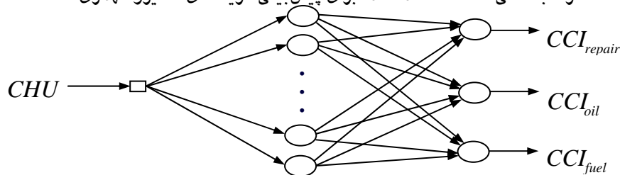
شکل (۲) ساختار شبکه کلی MLP استفاده شده برای پیش‌بینی هزینه‌های تعمیر و نگهداری
