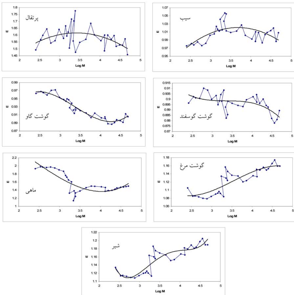
(شکل ۴) - رابطه کشش درآمدی از تابع AIDADS و درآمد سرانه (الگوی مقید)
