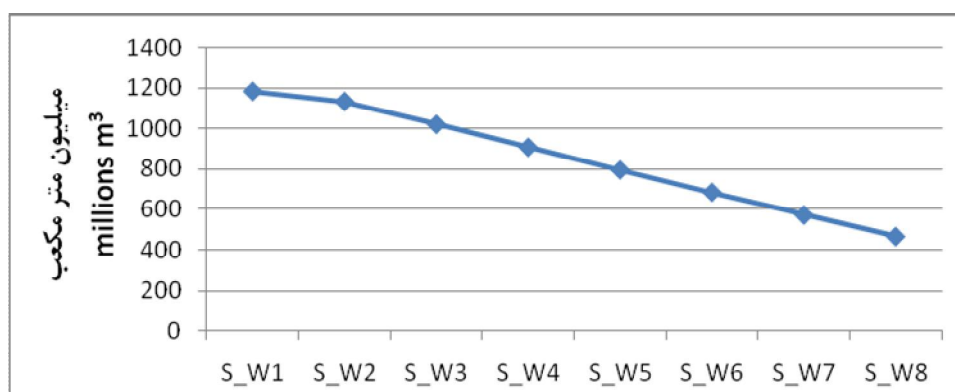
شکل 3- منحنی تقاضای آب زیرزمینی در دشت مهیار شمالی در طی سالهای شبیه سازی
