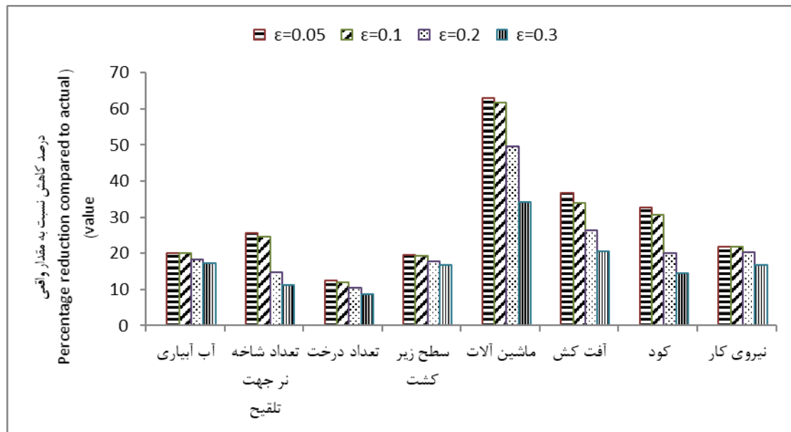
شکل ۲- درصد کاهش نهاده‌ها نسبت به مقدار واقعی در P=0.8 و سطوح اطمینان مختلف Figure 2- The percent reduction in inputs relative to the actual value at P = 0.8 and various confidence levels
